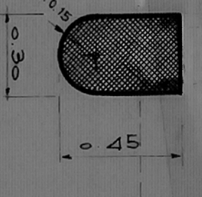
DÉTAIL POTEAUX B.A. PRÉAUX
